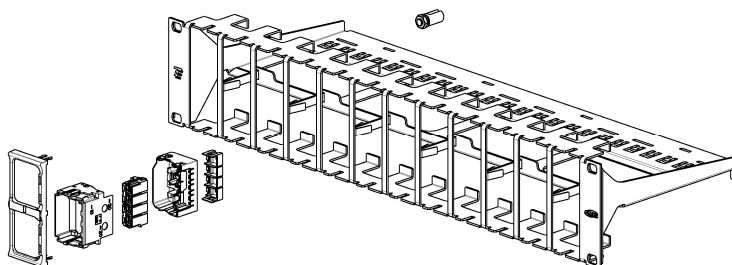
Rys.5 Ekranowany panel krosowy uniwersalny 24port 2GHz
