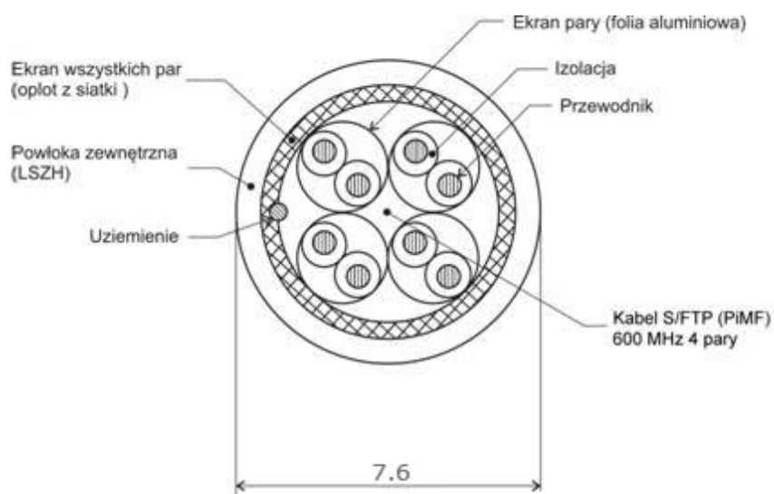
Rys. 4 Przekrój kabla S/FTP (PiMF) 600MHz
