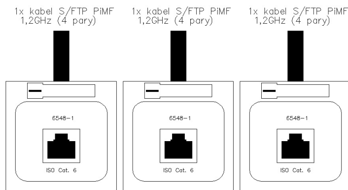
Rys. 3. Konfiguracja Punktu Logicznego.
